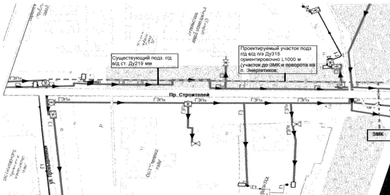
«Схема 305. Реконструкция подземного газопровода высокого давления в г. Энгельс по пр. Строителей от ул. Полтавской до пос. Энергетиков, инв. № 200226
