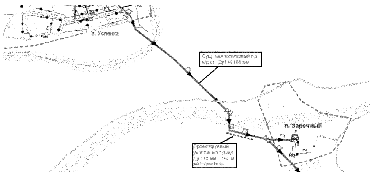
Схема 306. Реконструкция газопровода высокого давления в с. Успенка Пугачевского района (пансионат «Пугачевский»), инв. № 734 (2 этап)
